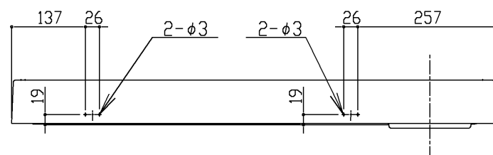
パン本体穴加工位置（現場加工）
