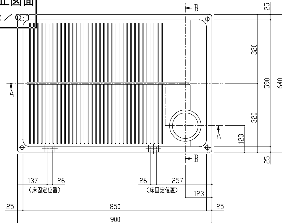
洗濯機設置有効寸法組合せ
